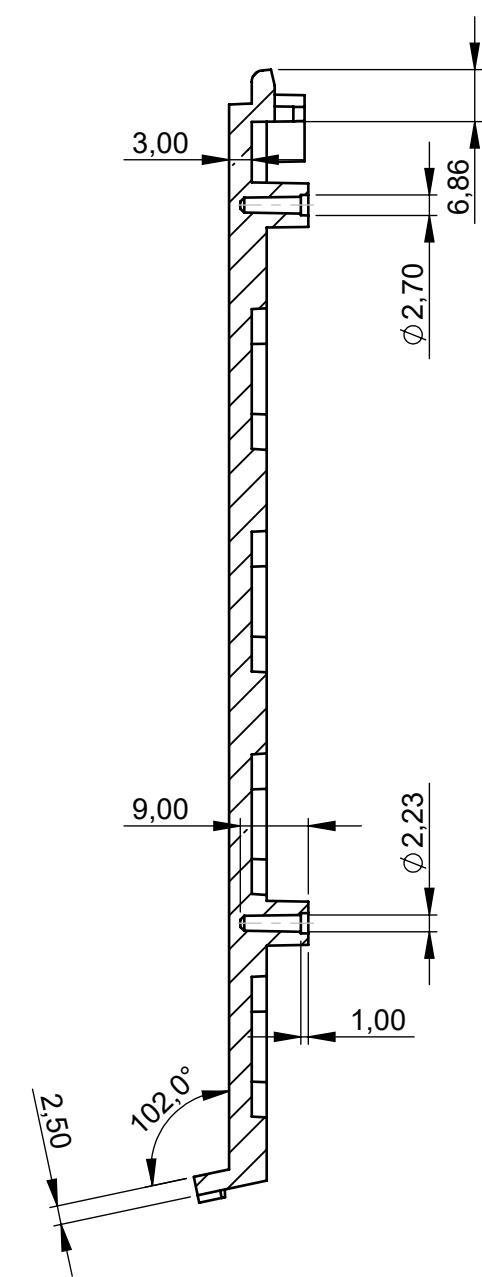
Schnitt A-A
