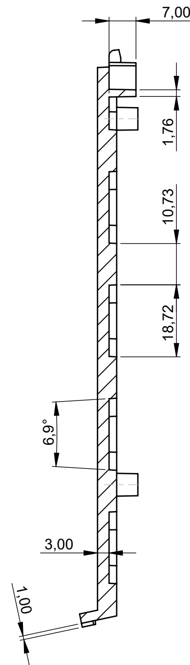
Schnitt B-B
