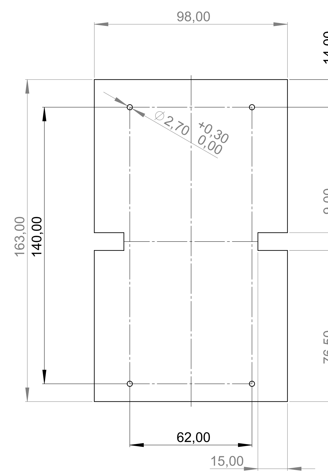
Platine Unterteil P C B Bottom Part
