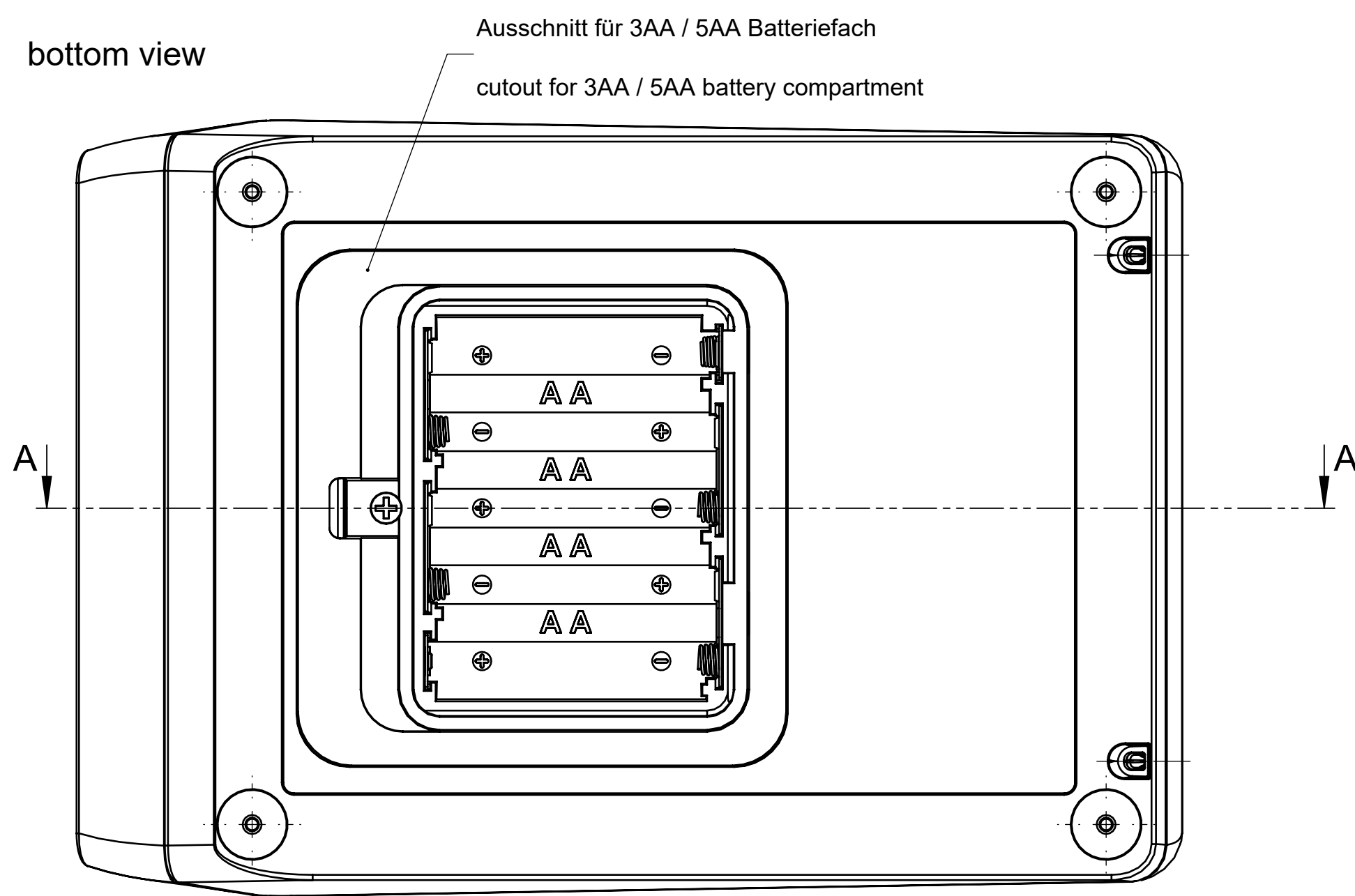
Hauptteil mit Batteriefach Main section with battery compartment
