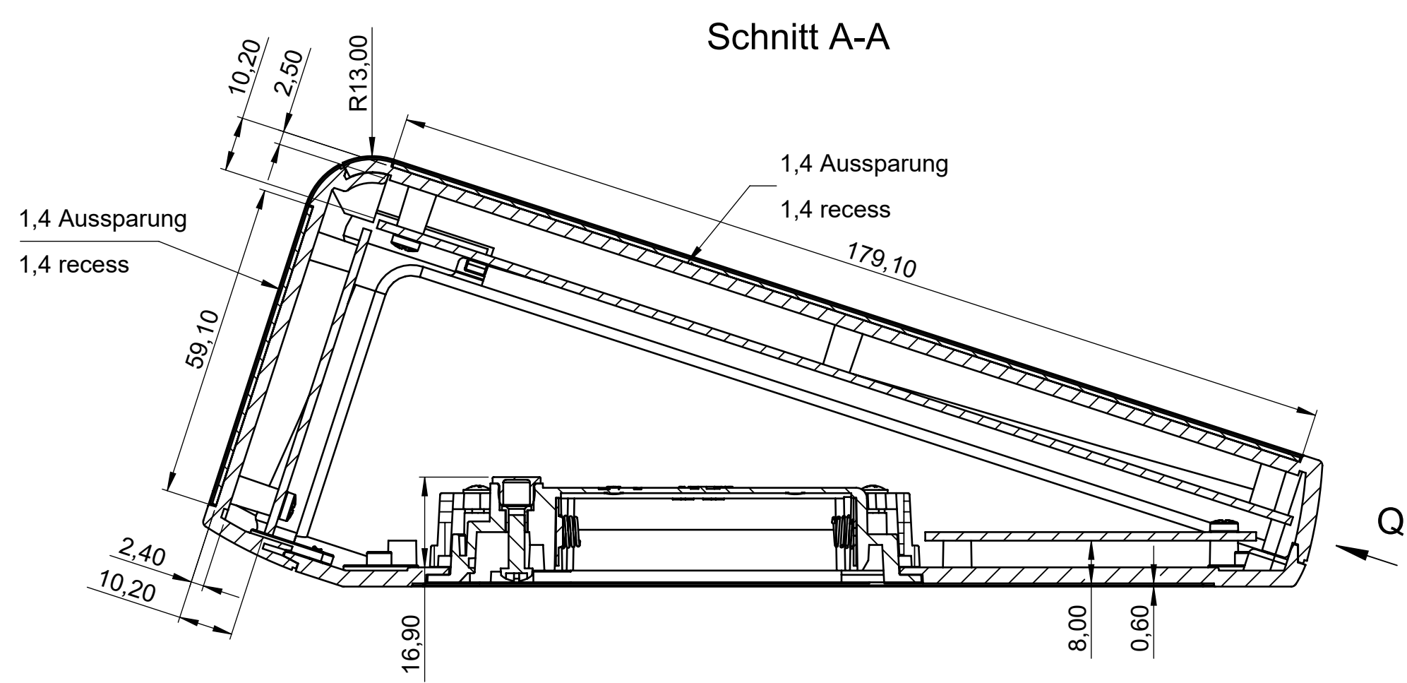
Schnitt A-A
