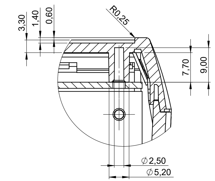
Detail Y (2 : 1)
