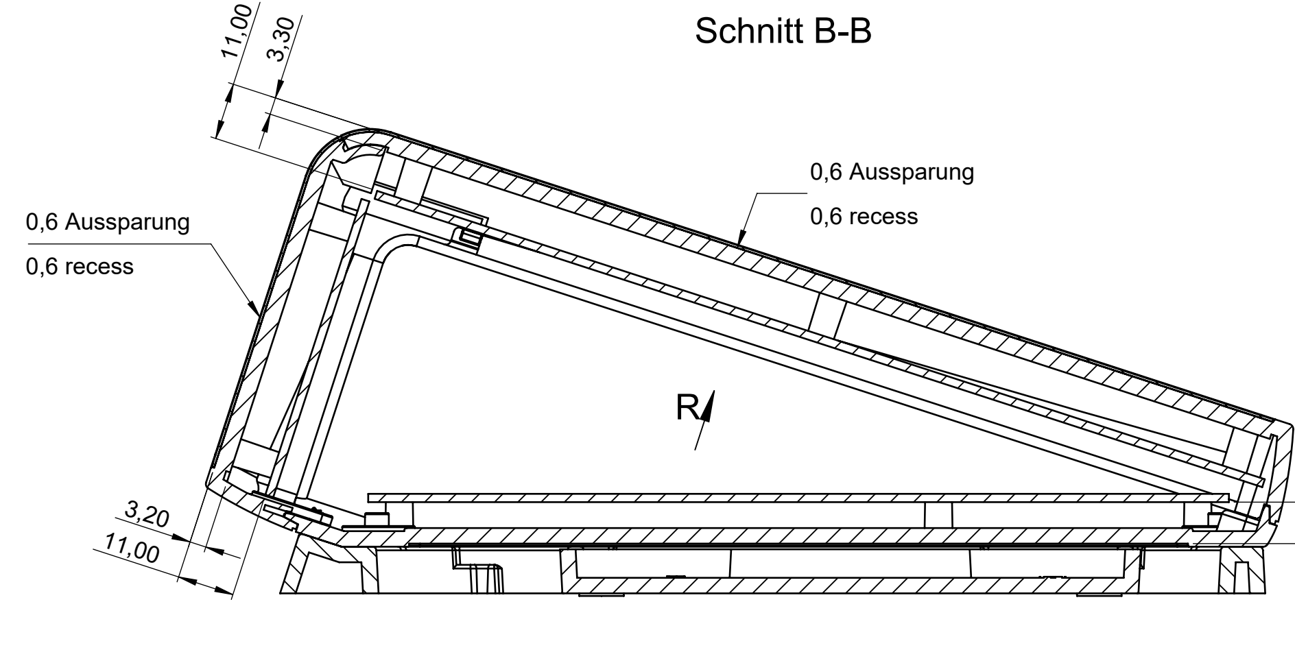
Schnitt B-B
