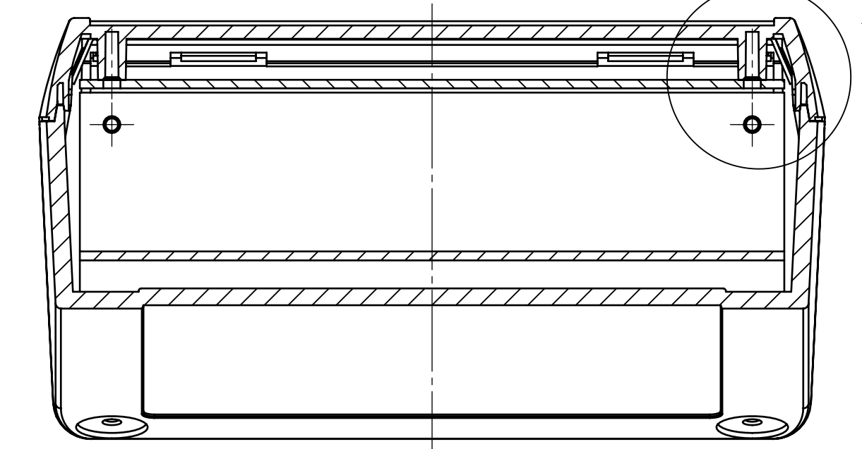
Schnitt N-N
