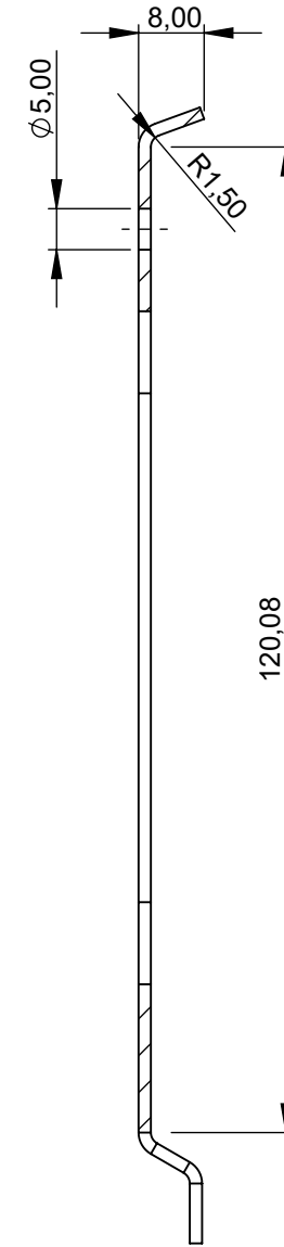
Schnitt B-B
