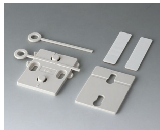
A9305017 Jeu de support mural ASA+PC-FR (UL 94 V-0) gris blanc RAL 9002
